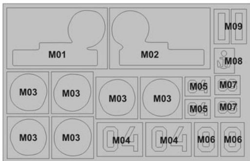
Расположение окрасочных масок, используемых для окраски моделей Су-24М ВКС России в Сирии.
