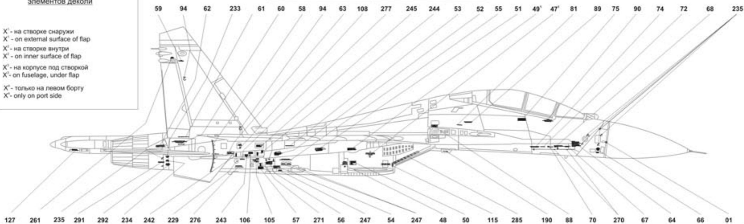
Су-27УБ поздних (с 10-ой серии) производственных серий, вид слева
