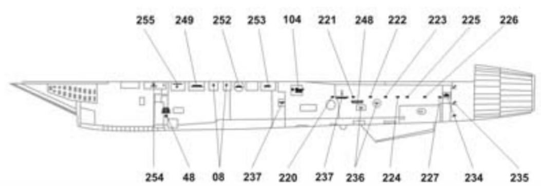
Су-27 всех производственных серий, внутренняя сторона левого киля Su-27 from all productional batches, inner surface of port side fin
