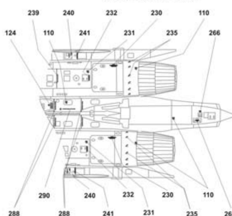
Су-27 с 18-ой и Су-27УБ с 10-ой (поздние производственные серии), хвостовая часть, вид снизу Su-27 after 18-th batch and Su-27UB after 10-th productional batch, bottom view of fuselage tail section
