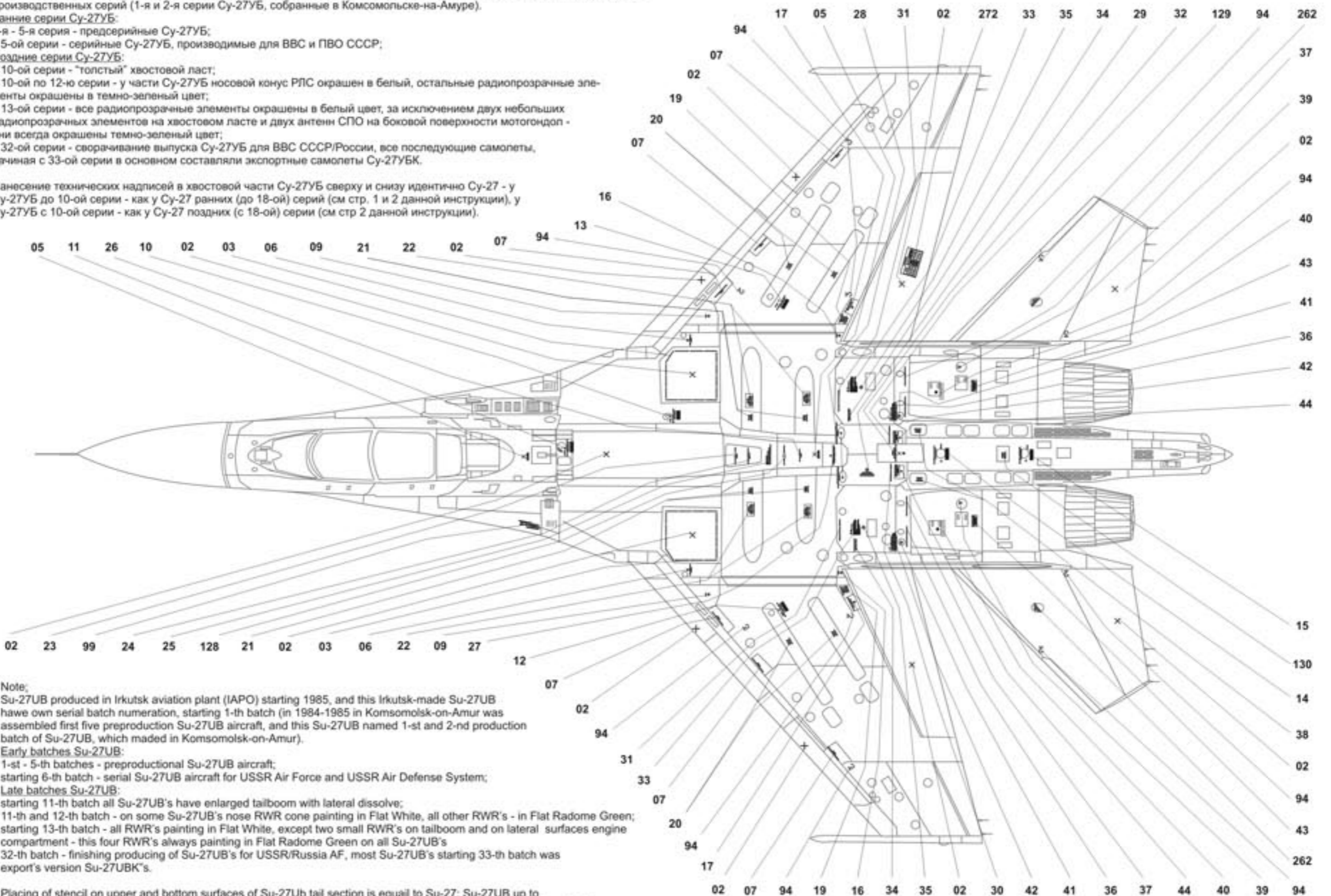
Су-27УБ поздних (с 10-ой серии) производственных серий, вид сверху Su-27UB from late, after 10-th production batch, top view
